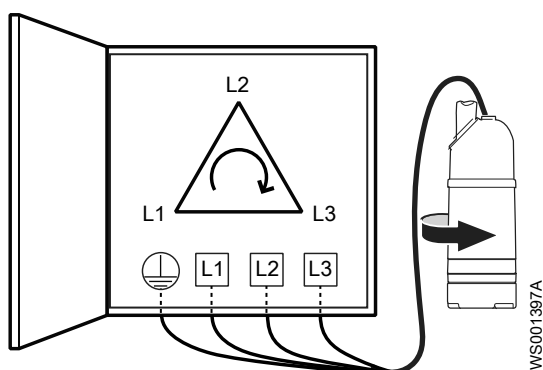
Рис. 3: Включите насос
