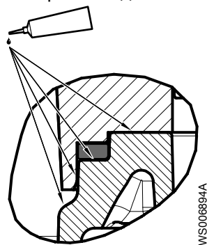
Рис. 4: Пример сопрягаемых поверхностей уплотнительного кольца
