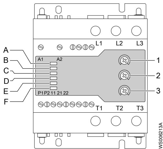
Рис. 7: Разводка клемм устройства плавного пуска
